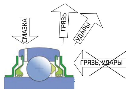
Уплотнение 2ТВ
